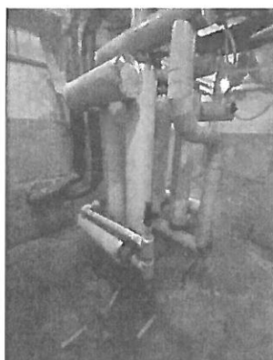
Fot. 3.2. Przykład węzła z rurkowym typu JAD, dwustopniowym wymiennikiem przepływowym.
